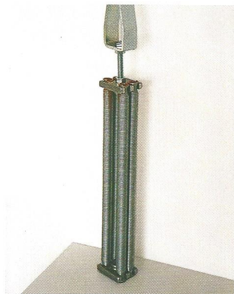
Federpakete für normale Tore maximal 4 Einzelfedern
